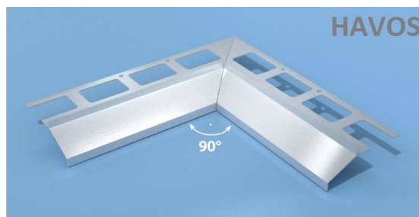
Roh k okapnicovému profilu 40 mm- vnitřní
